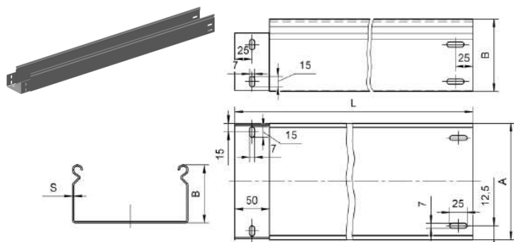
ЛМС-ПЗНМ
