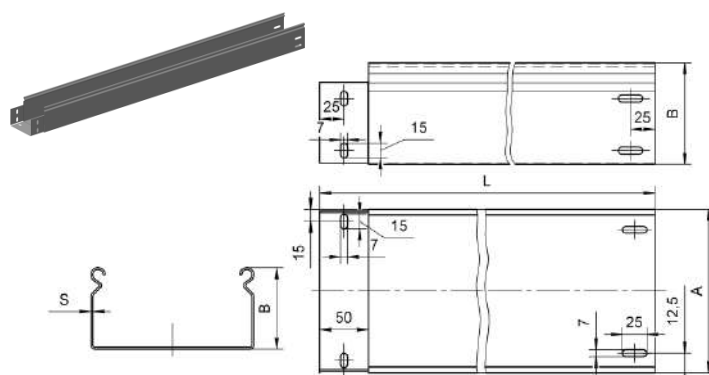
ЛМС- ПЗНМ
