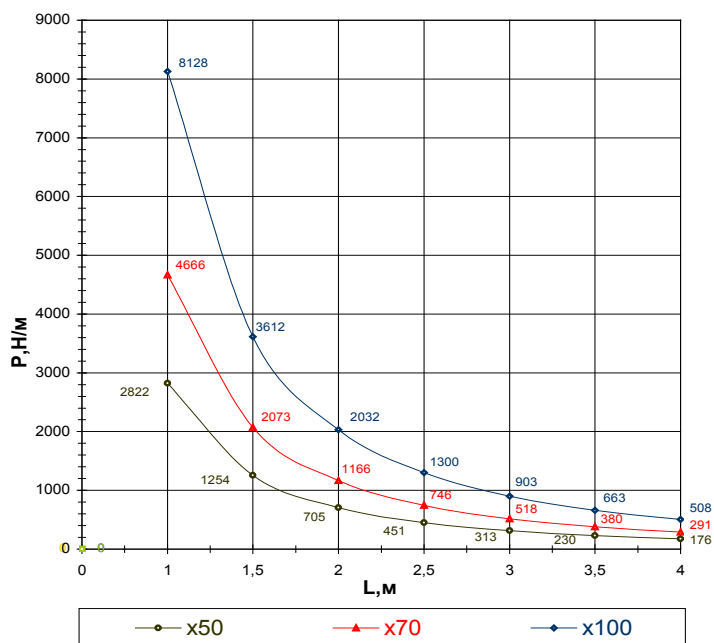
Лоток НЛ20(30,40)-1,5
