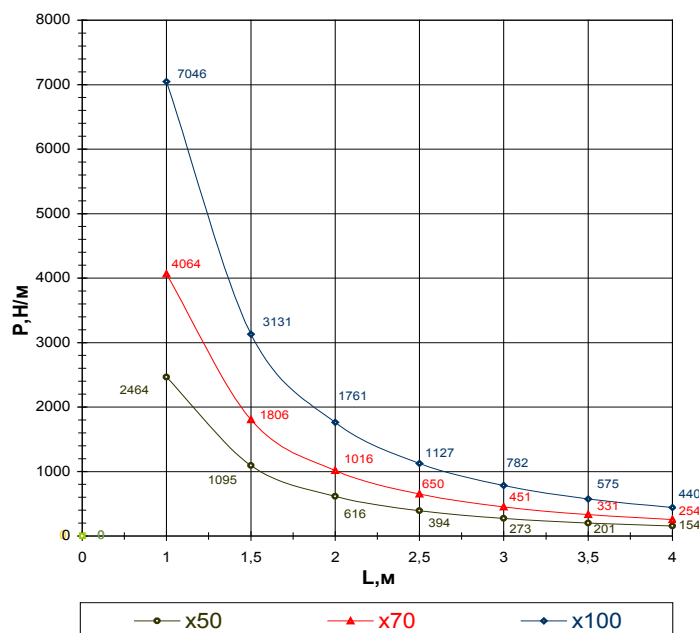
Лоток НЛ20(30,40)-1,2
