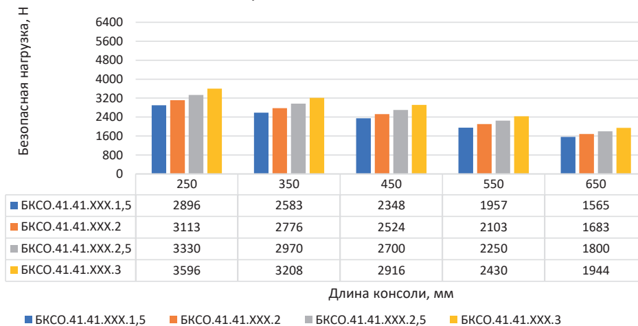
Консоль страт облегченная БКСО, ширина 41 мм, высота 41 мм
