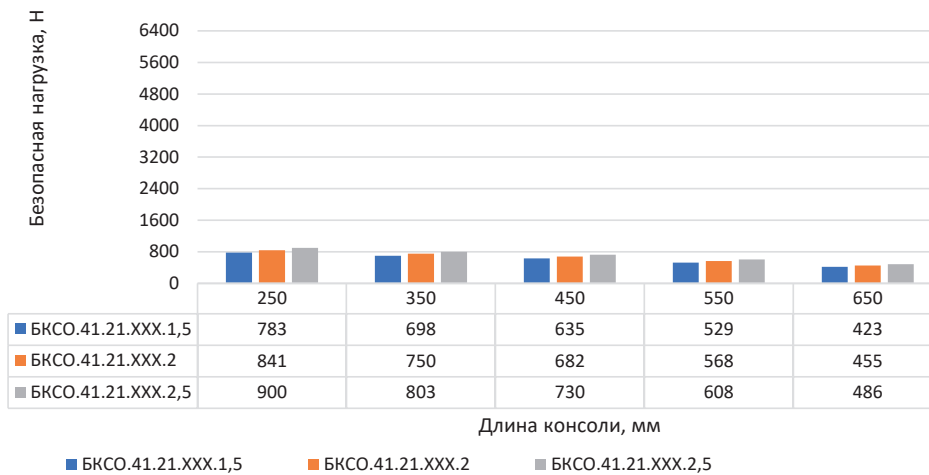
Консоль страт облегченная БКСО, ширина 41 мм, высота 21 мм
