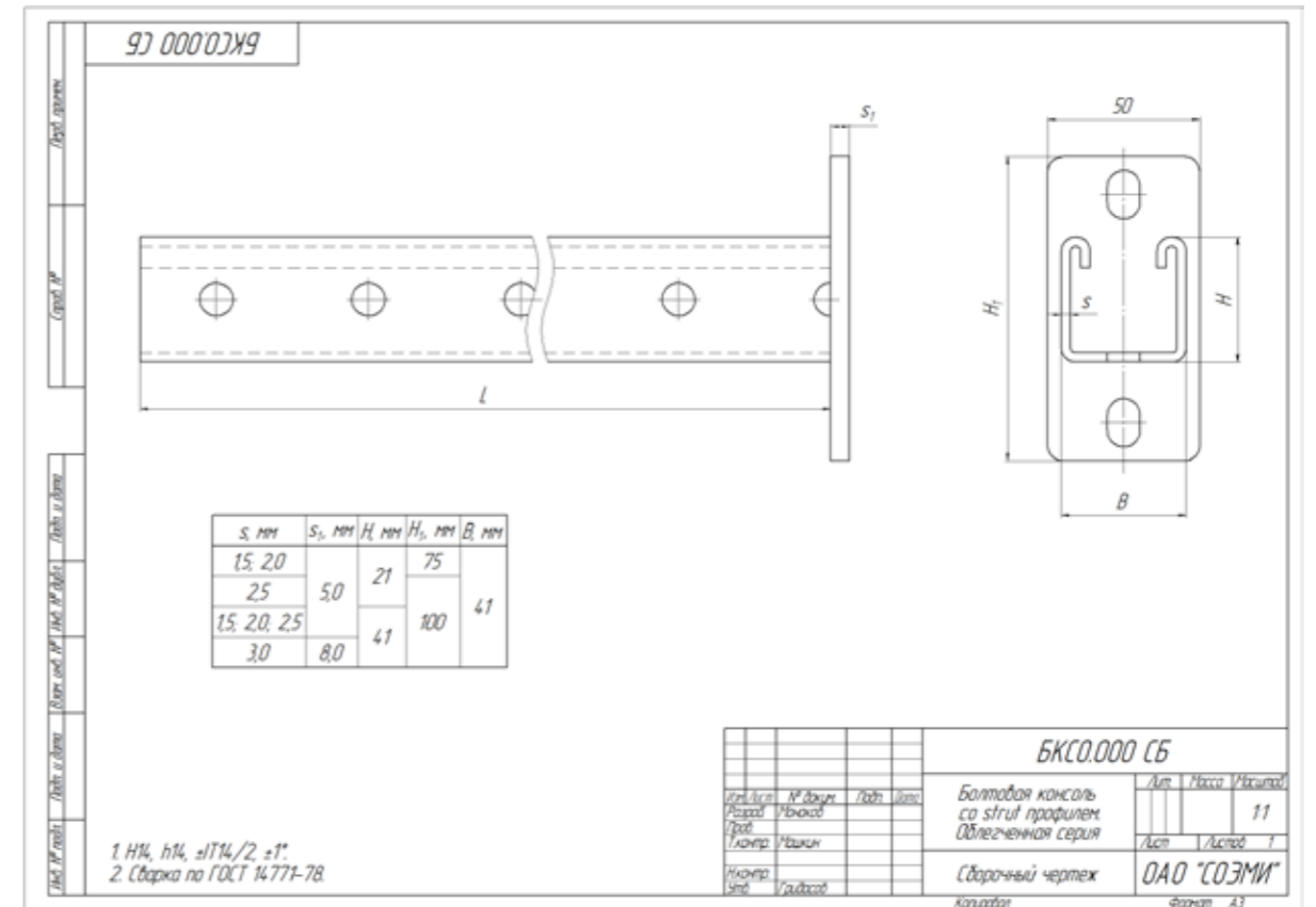
Консоль страт облегченная БКСО, ширина 41 мм, высота 21 мм
