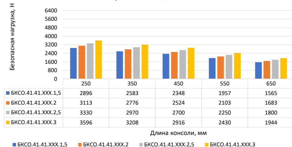
Консоль страт облегченная БКСО, ширина 41 мм, высота 41 мм
