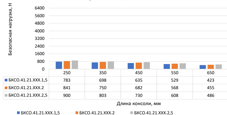
Консоль страт облегченная БКСО, ширина 41 мм, высота 21 мм
