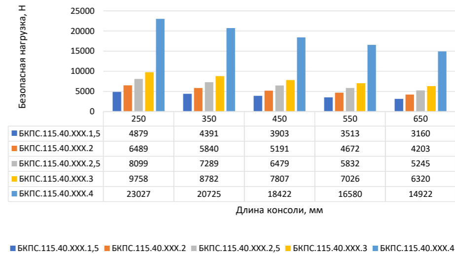
Консоль П - образная средняя БКПС, ширина 115 мм, высота 40 мм
