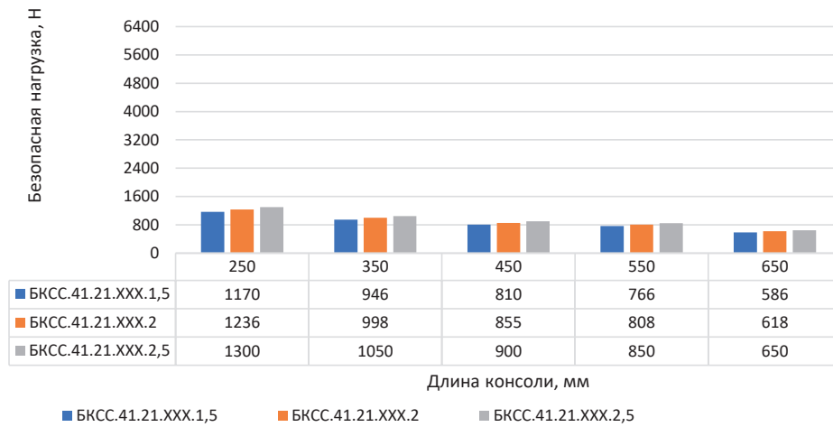
Консоль страт средняя БКСС, ширина 41 мм, высота 21 мм
