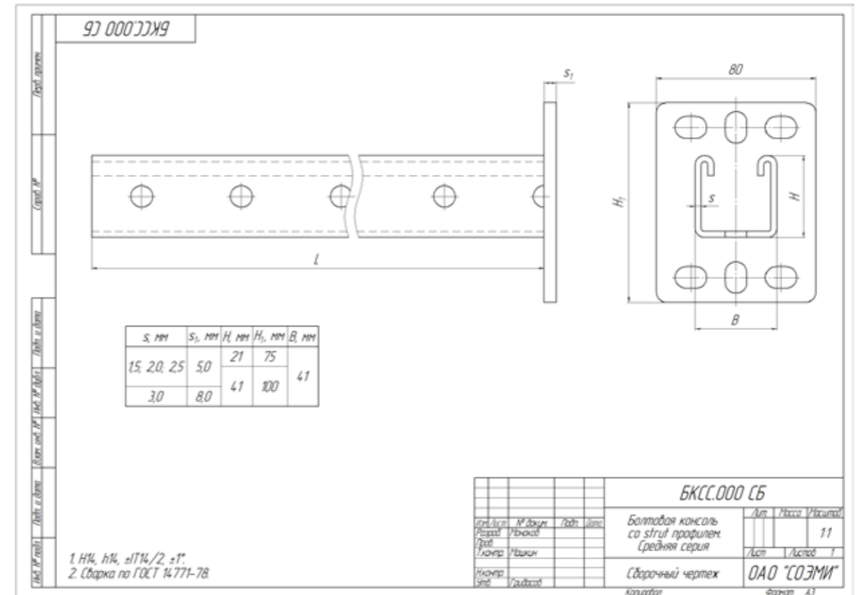
Консоль страт средняя БКСС, ширина 41 мм, высота 21 мм
