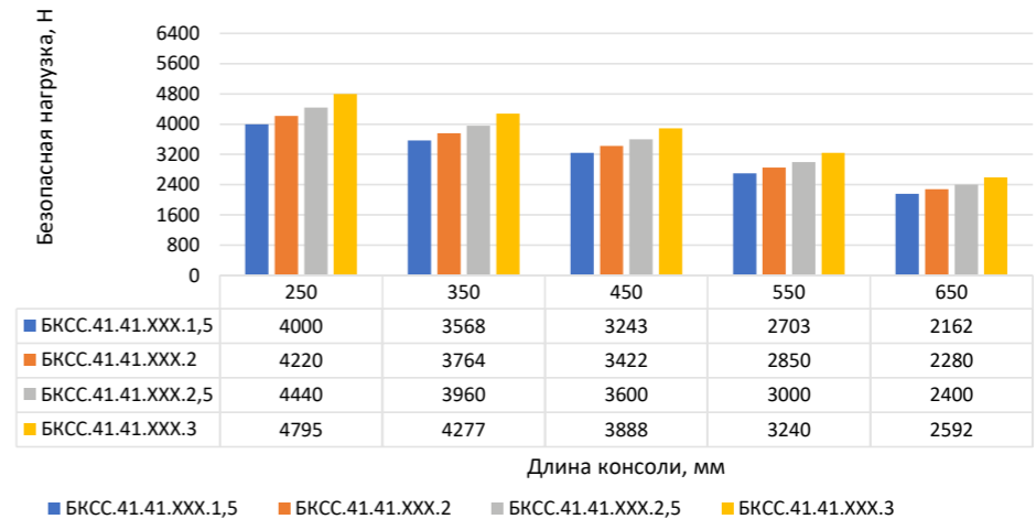
Консоль страт средняя БКСС, ширина 41 мм, высота 41 мм
