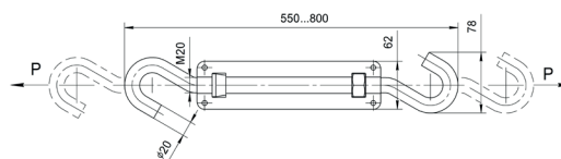
Муфта K805
