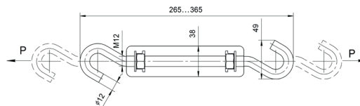
Муфта K804M
