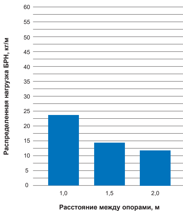
Лоток проволочный ППУ5, борт 60 мм
