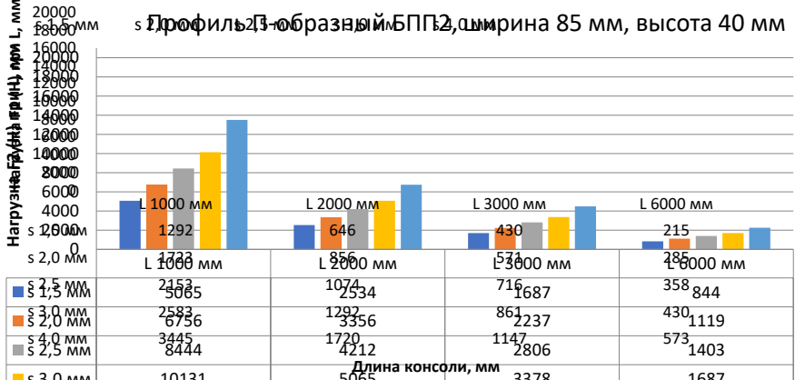
Профиль П - образный БПП2, ширина 115 мм, высота 40 мм
