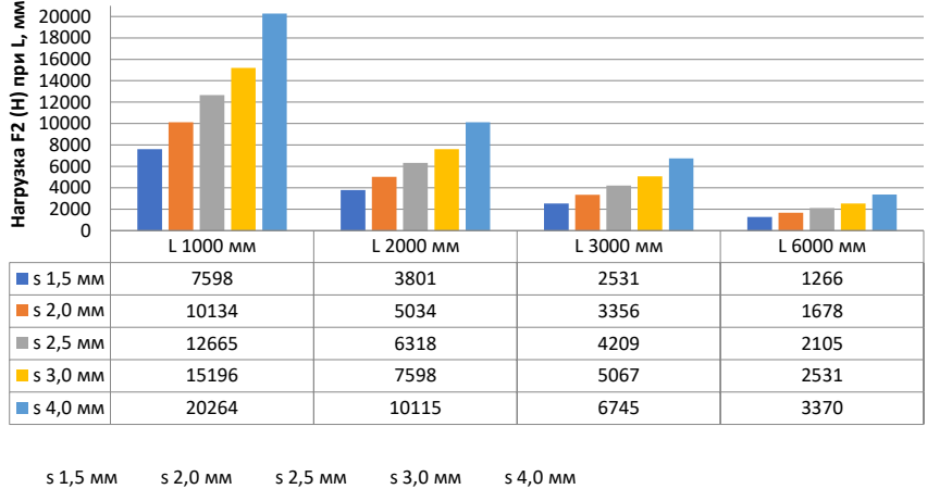
Профиль П-образный БПП2, ширина 115 мм, высота 40 мм
